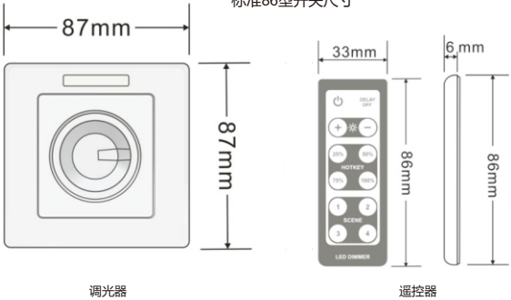
标准86型开关尺寸
